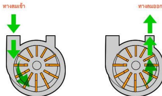
ภาพที่ 4 ปั๊มลมแบบใบพัดเลื่อน
