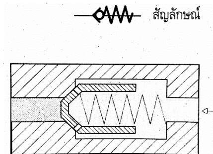
ภาพที่ 24 วาล์วกั้นกลับทางเดียวพร้อมสัญลักษณ์
