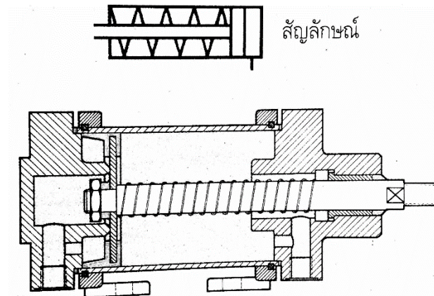
ภาพที่ 37 กระบอกลมทำงานด้านเดียว พร้อมสัญลักษณ์
