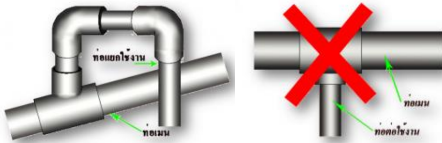
ภาพที่ 18 การต่อท่อแยกด้วยข้ออฉาก
