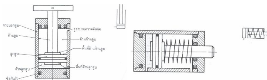
กระบอกสูบทางเดียวใช้แรงจากภายนอกเลื่อนลูกสูบกลับ กระบอกสูบทางเดียวใช้สปริงเลื่อนลูกสูบกลับ ภาพที่ 21 กระบอกสูบทางเดียว พร้อมสัญลักษณ์
