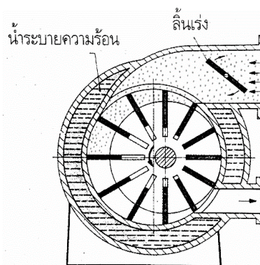
ภาพที่ 5 ปั๊มไฮดรอลิกส์แบบเวน
