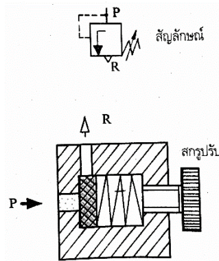
ภาพที่ 28 วาล์วจำกัดความดันลดพร้อมสัญลักษณ์
