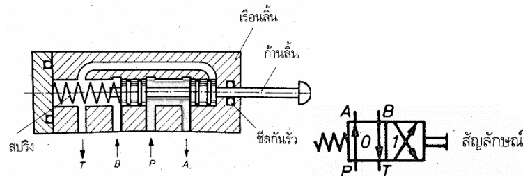
ภาพที่ 11 วาล์วทิศทาง 4/2 แบบปุ่มกดปกติปิด พร้อมสัญลักษณ์
