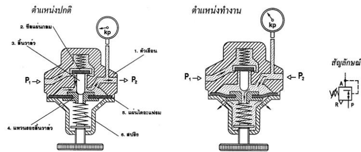
ภาพที่ 12 ตัวปรับความดันลดพร้อมสัญลักษณ์
