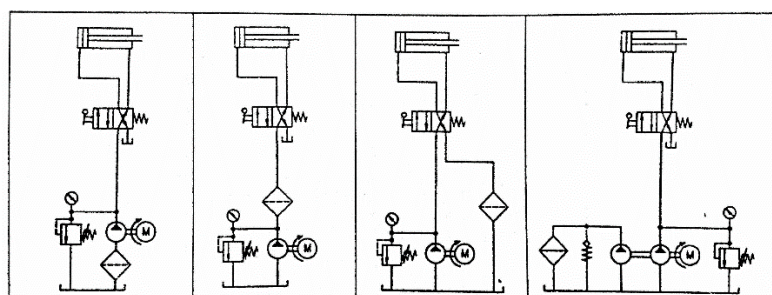
ภาพที่ 24 ตำแหน่งการกรองน้ำมันไฮดรอลิกส์
