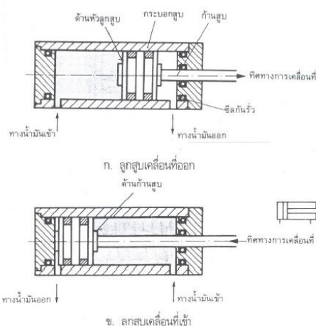
ภาพที่ 22 กระบอกสูบสองทาง พร้อมสัญลักษณ์
