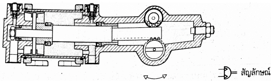
ภาพที่ 39 กระจบบกลแบบส่งแรงหมุน พร้อมสัญลักษณ์
