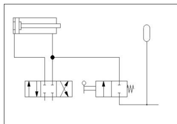
.....วงจรที่ 1 เมื่อพลังงานหลักหยุดทำงาน สามารถใช้แรงดันจาก Accumulator
