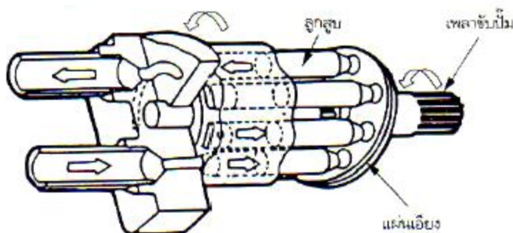
ภาพที่ 7 ปัมไฮดรอลิกส์แบบลูกสูบชนิดลูกสูบอยู่แนวเดียวกับแกนเพลลา
