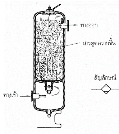
ภาพที่ 10 ตัวกรองความดันลดด้วยการดูดซึมพร้อมสัญลักษณ์
