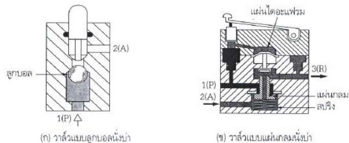
ภาพที่ 19 วาล์วควบคุมทิศทางการไหลต่างๆ
