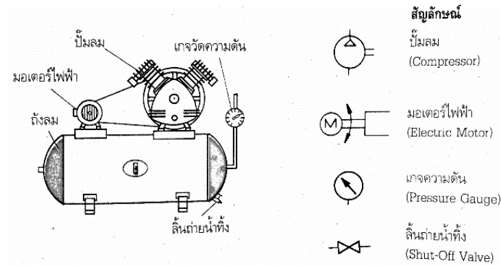
ภาพที่ 1 ชุดต้นกำลังนิวเมติกส์และสัญลักษณ์พื้นฐาน
