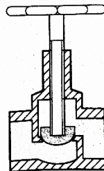
ภาพที่ 35 วาล์วเปิด-ปิด ลม พร้อมสัญลักษณ์
